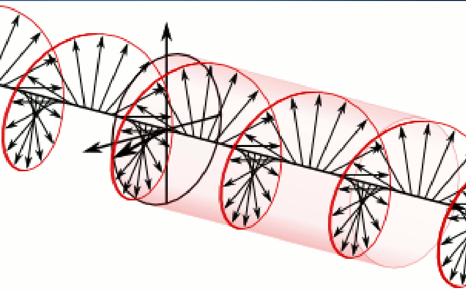
Polarización circular derecha (u horaria)
