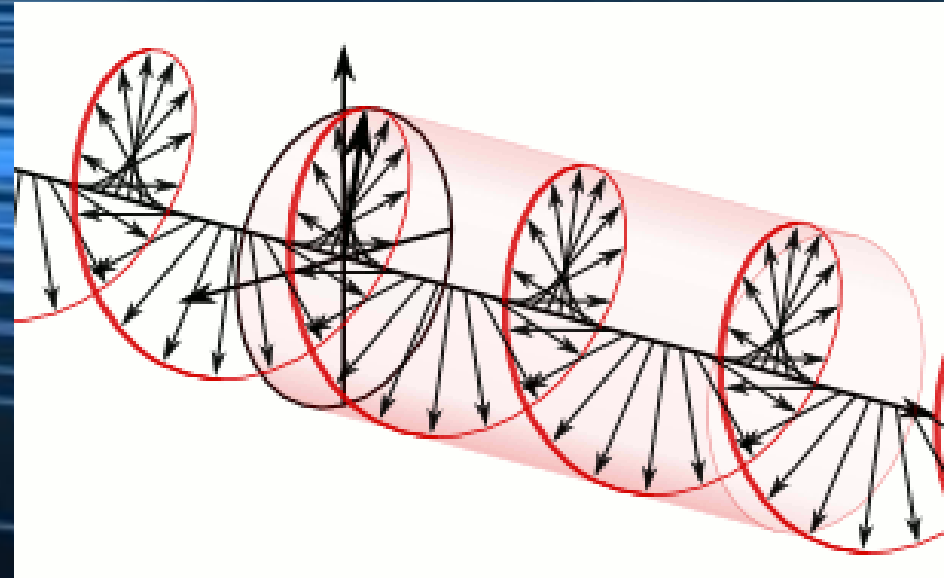
Polarización circular izquierda (o anti-horaria)
